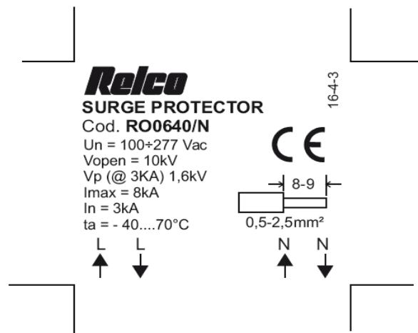
Limitatore di sovratensione - Surge protector
