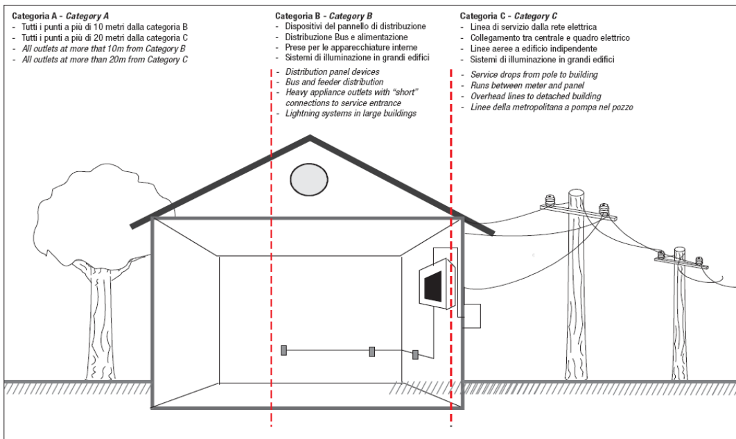
IEE C62.41 - Forme d'onda di corrente / tensione per varie località di esposizione - Current/Voltage waveforms for various exposure locations
