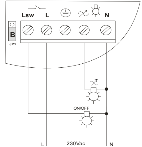
B JP2 posizione "B" Funzionamento due fonti luminose 1) ON/OFF 2) REGOLAZIONE
