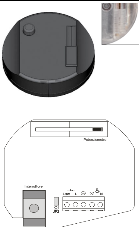
A JP2 posizione "A" Funzionamento una fonte luminosa 1) ON/OFF e REGOLAZIONE
