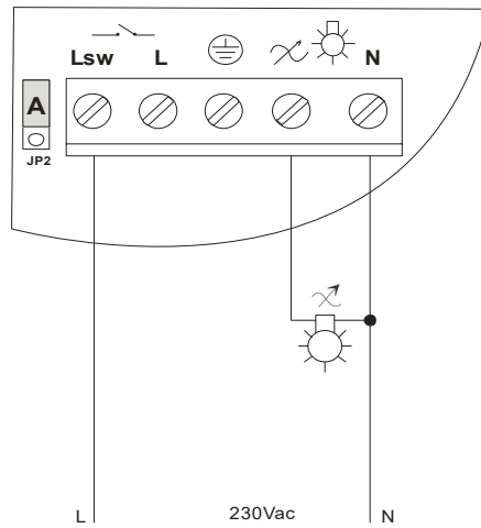
A JP2 posizione "A" Funzionamento una fonte luminosa 1) ON/OFF e REGOLAZIONE
