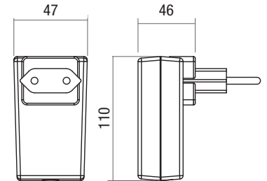
Dimensioni (mm) - Dimensions (mm)
