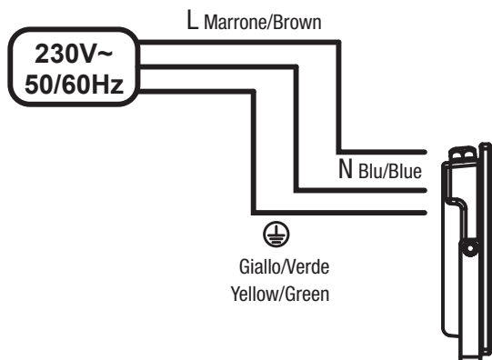
Fig. 9 Schema di collegamento in serie Serie connection diagram
