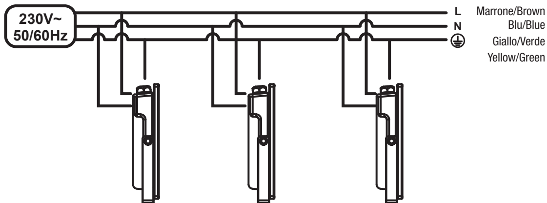
Fig. 8 Schema di collegamento in parallelo Parallel connection diagram
