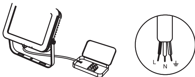
Fig. 5 Collegare il cavo di alimentazione - Plug in the power wire
