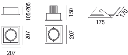
Dimensioni - Dimension (mm)
