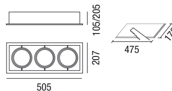
Dimensioni - Dimension (mm)
