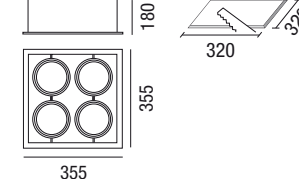
Dimensioni - Dimension (mm)
