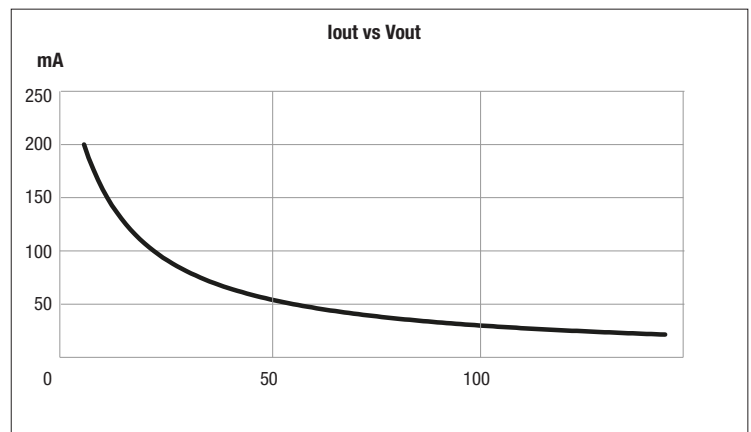
Fig. 1 - Caratteristica tensione / corrente - Output characteristic voltage / current
