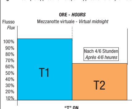
Fig. 1 - Esempio applicativo 2 steps - Application example 2 steps
