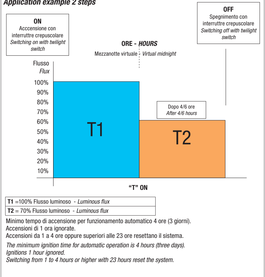
Fig. 1 - Esempio applicativo 2 steps Application example 2 steps
